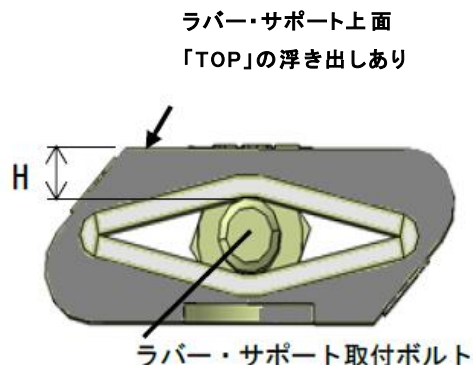
第14図. ラバー・サポート点検
