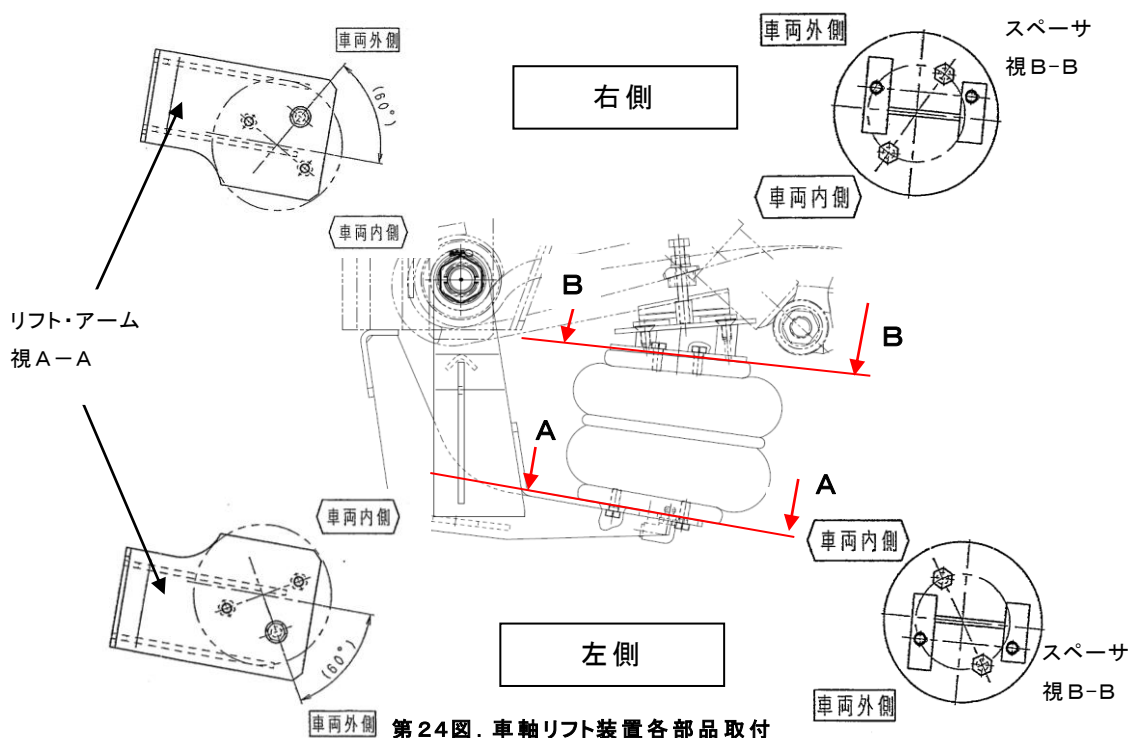
第24図. 車軸リフト装置各部品取付
