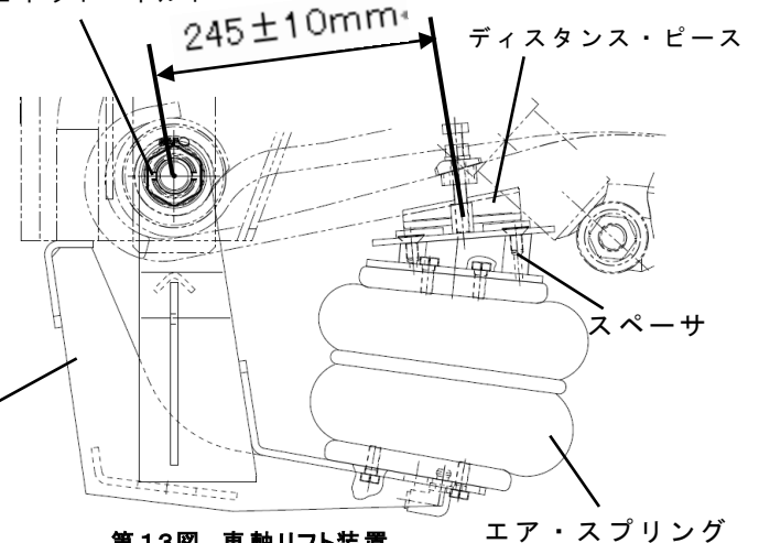
第13図. 車軸リフト装置
