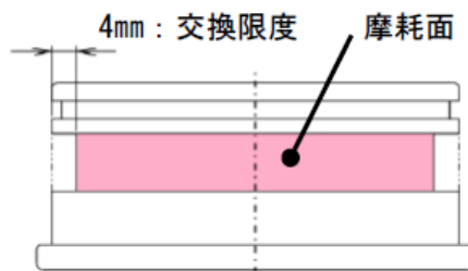
第15図. ガタの点検
