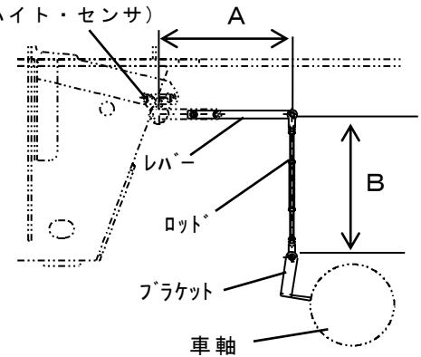
第4図. レバー、ロッドの長さ計測
